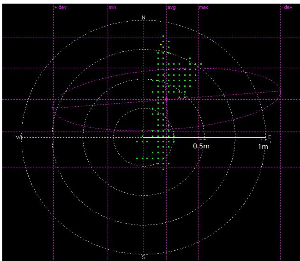
图 1 静态测试漂移轨迹图
